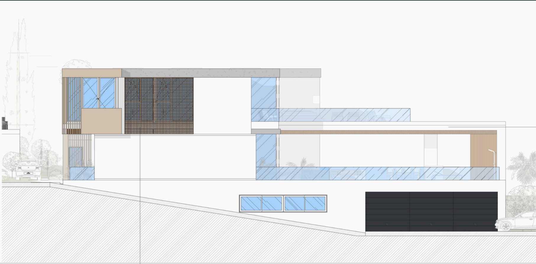
ALZADO OESTE
